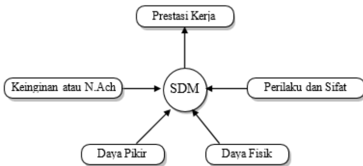
Gambar 2. Konsep SDM
